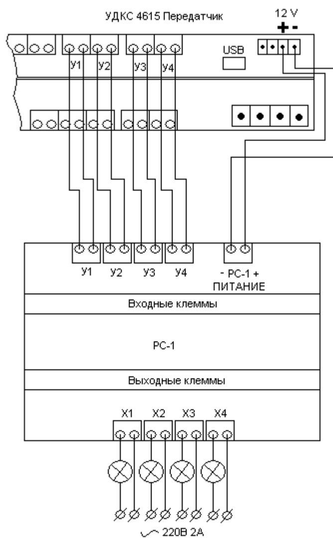
Схема подключения реле сопряжения РС-1
