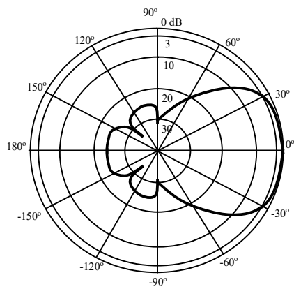
Диаграммы направленности антенны АН-433 в Е -плоскости и Н-плоскости
