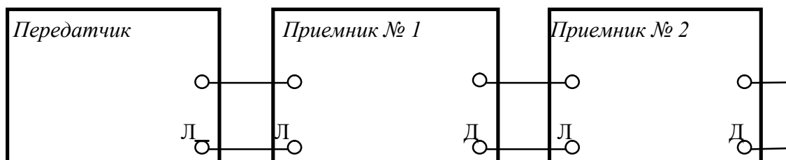
Рис.9 Схема соединения передатчика с приемниками в системе УДКС 4615 – 01.
