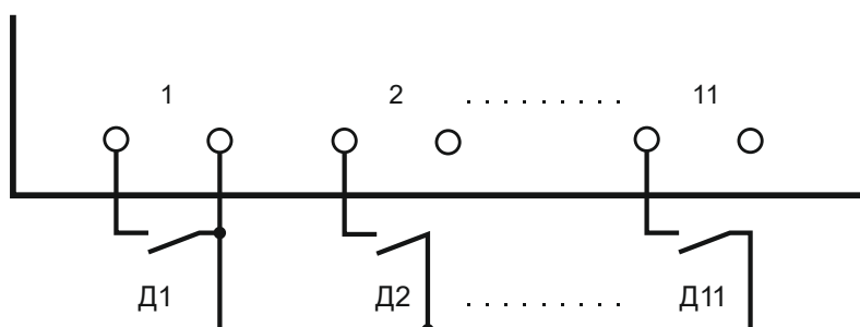
б) Датчики имеющие общий провод.
