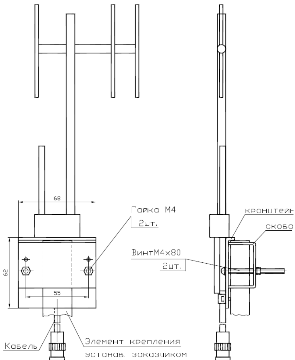
Чертёж узла крепления АН-433/Полярис-800-7
