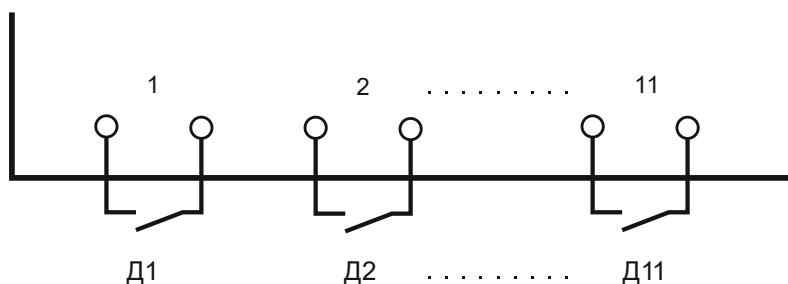
а) Датчики не имеющие общего провода.
