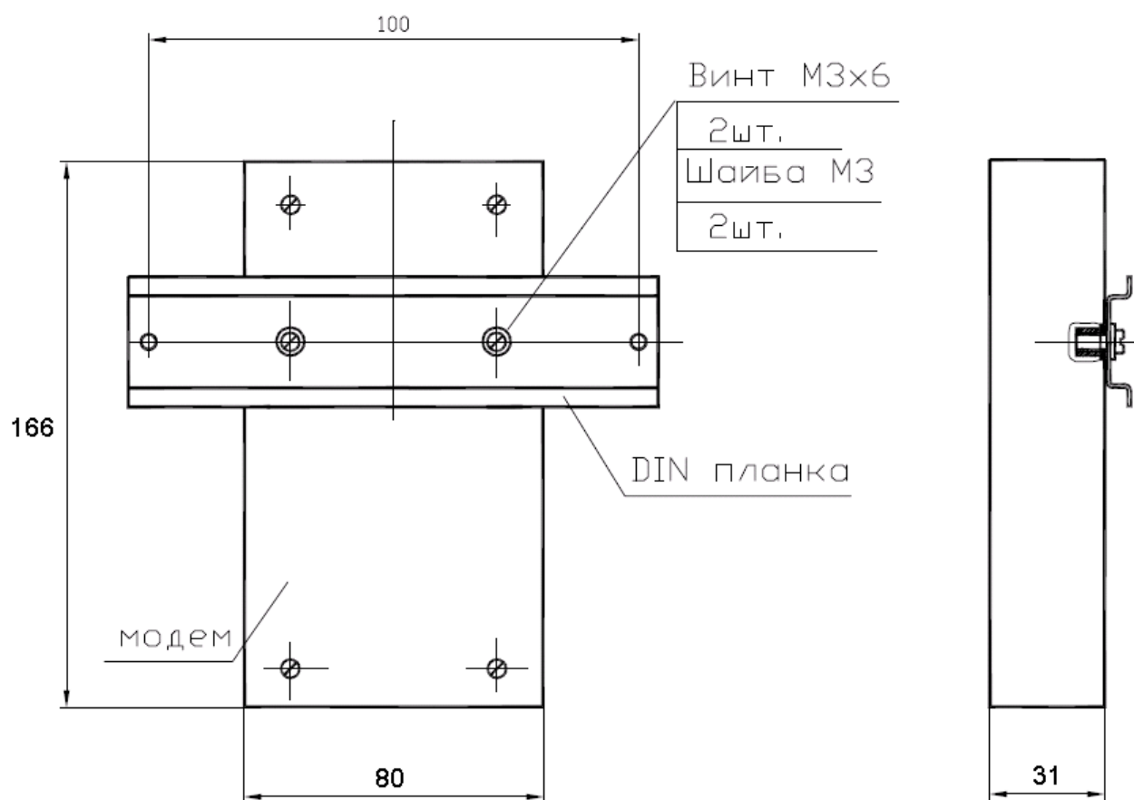
Чертеж узла крепления PM4615
