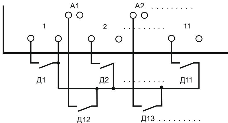
б) Расширение числа дискретных датчиков за счет аналоговых каналов
