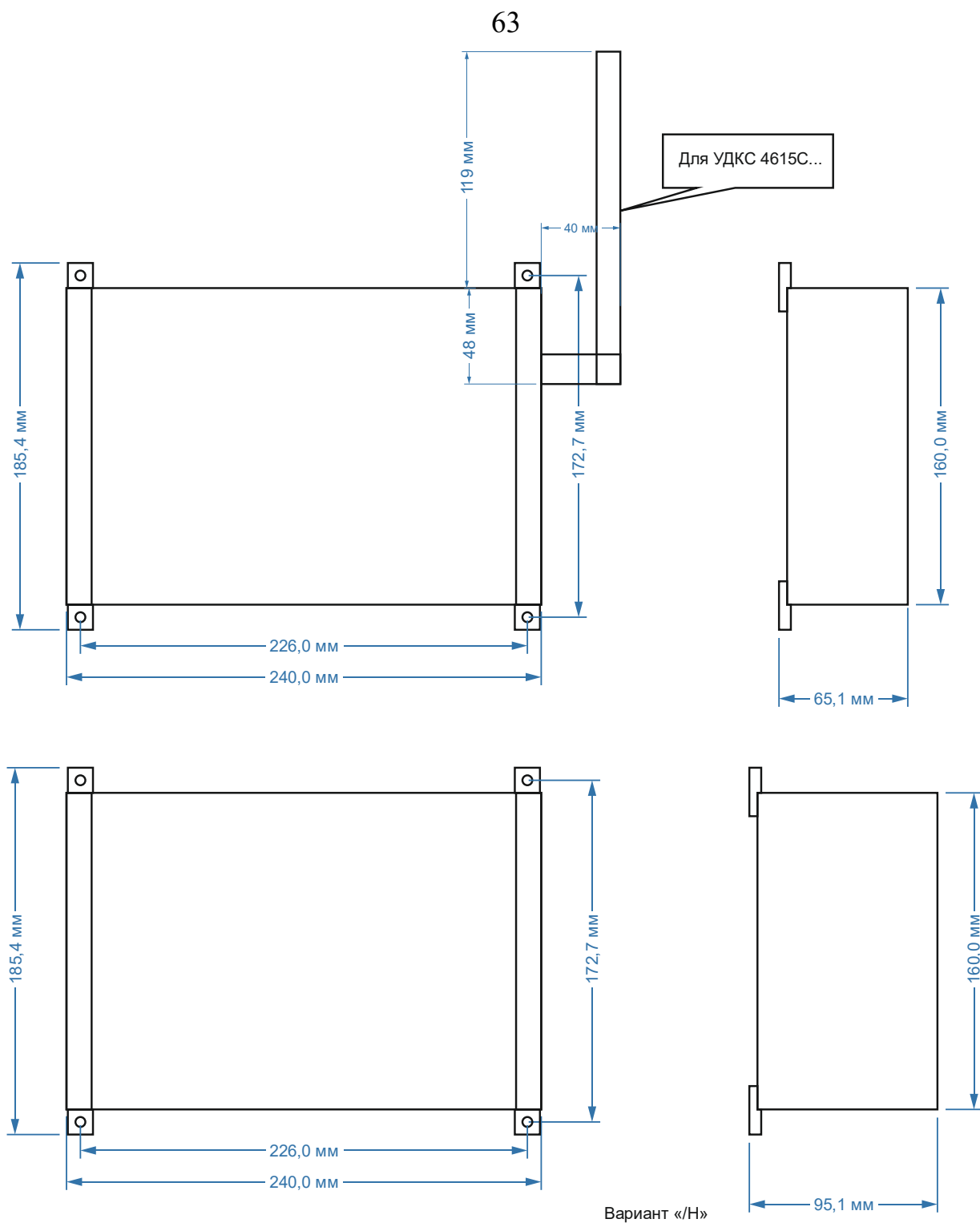
Рис.6 Габаритные размеры устройств.
