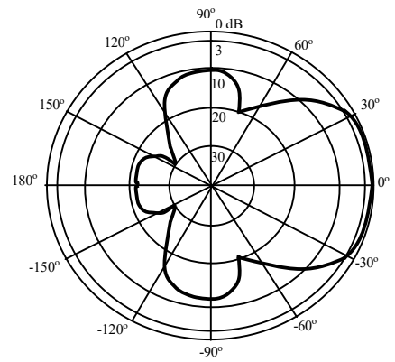
Диаграммы направленности антенны АН-433 в Е -плоскости и Н-плоскости
